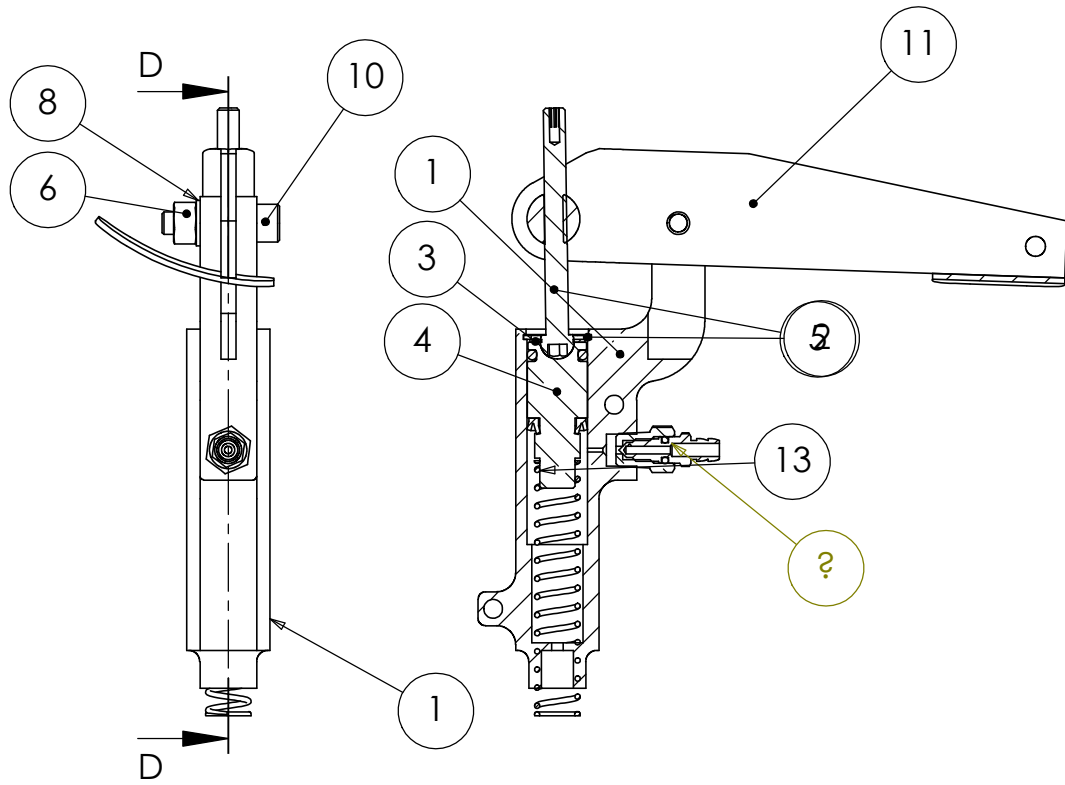
SEZIONE D-D
