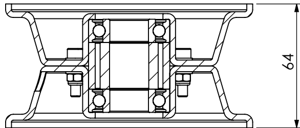
SEZIONE A-A SCALA 1 : 2
